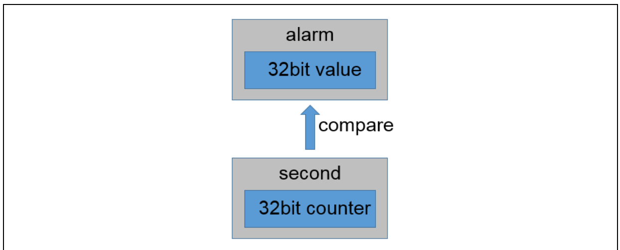
图 4. 闹钟匹配
