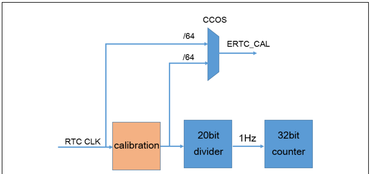
图 6. RTC 校准
