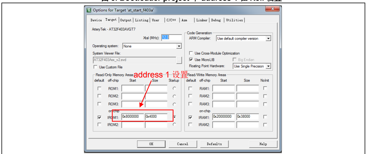
图 5. Bootloader project 中 address 1 在 Keil 设置
