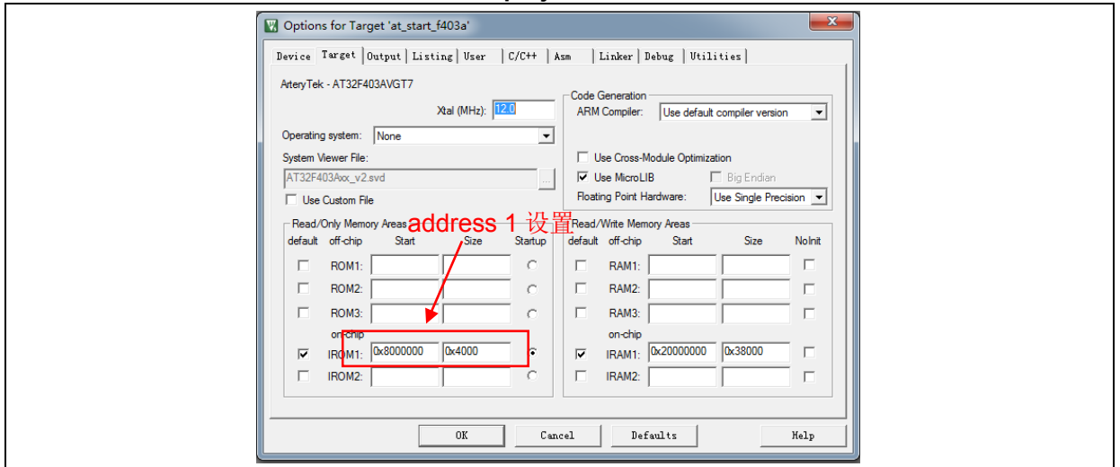
图 11. Bootloader project 中 address 1 在 Keil 设置
