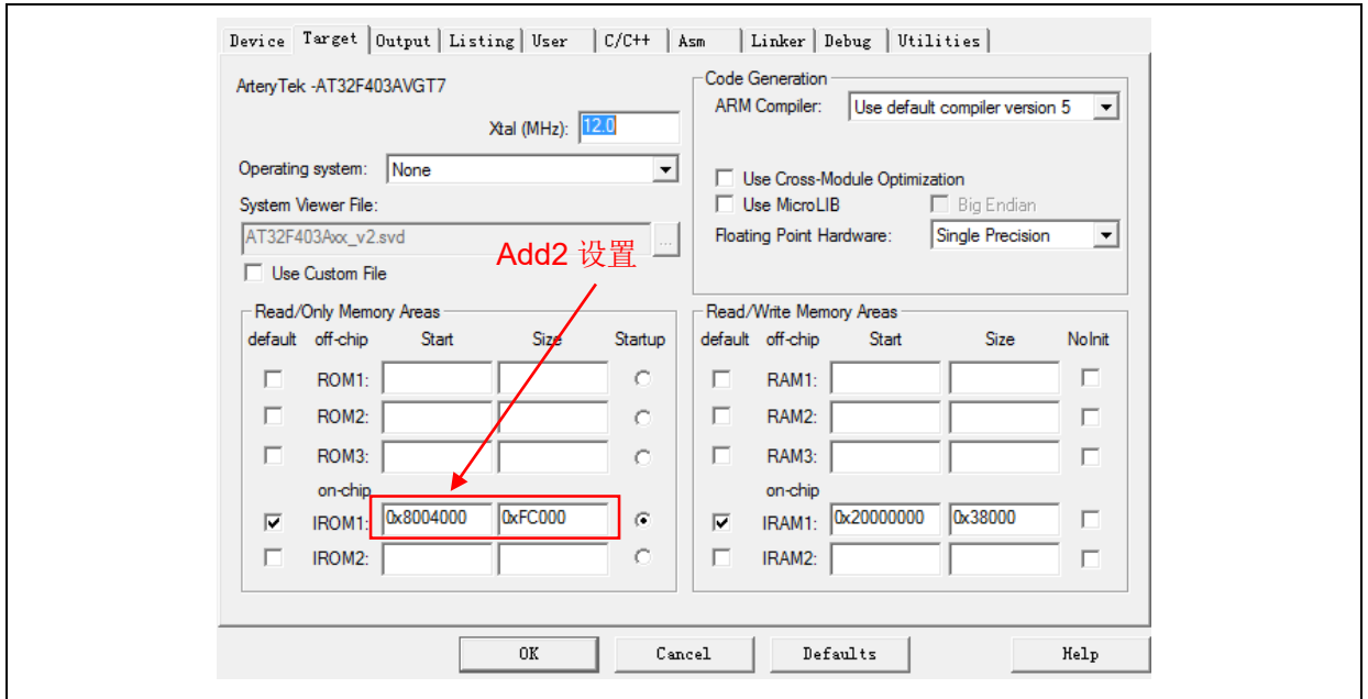
图 5. app project 中 add2 在 Keil 设置
