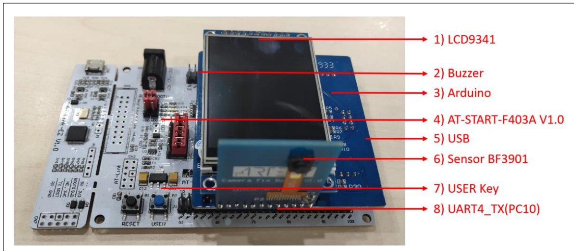
图 3. sensor board V1.0 硬件资源图
