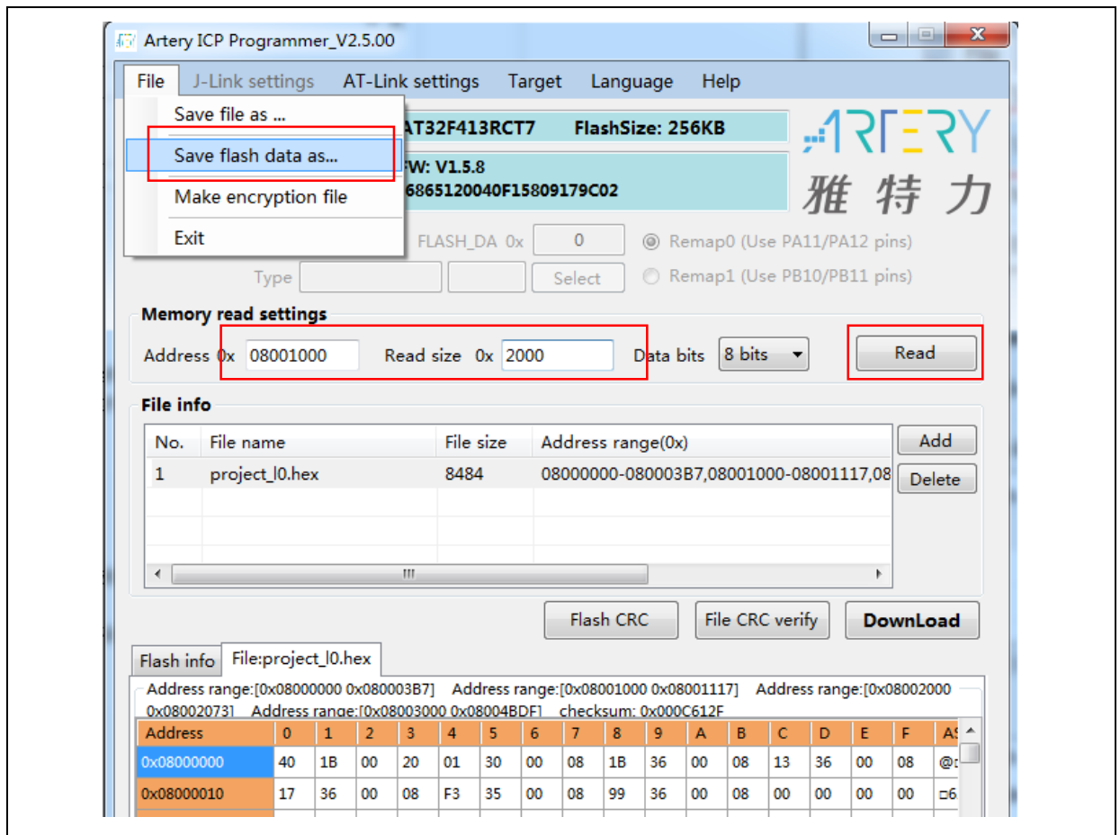
图 42. 保存 SLIB 代码
