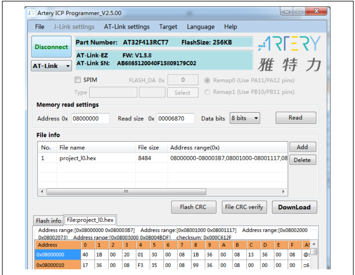
图 22. 配置 ICP Programmer
