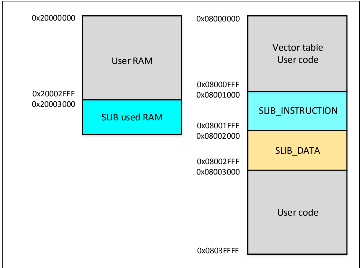
图 13. 范例程序的主闪存映像及 RAM 分区
