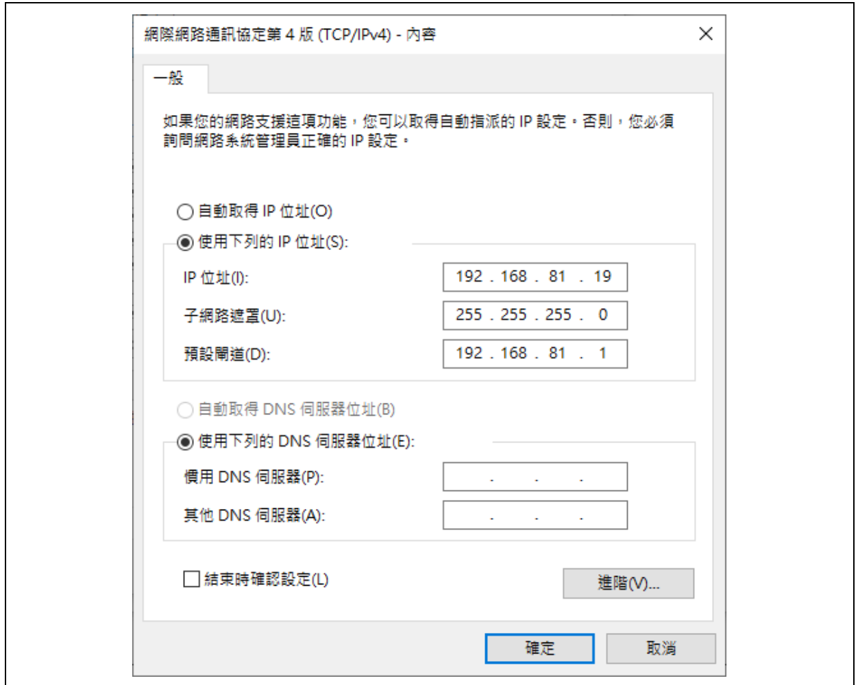
图 3. 设置 PC 端的 IP、网络屏蔽及网关
