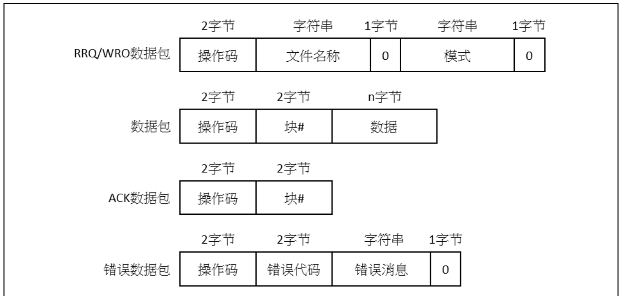
图 2 TFTP 数据包
