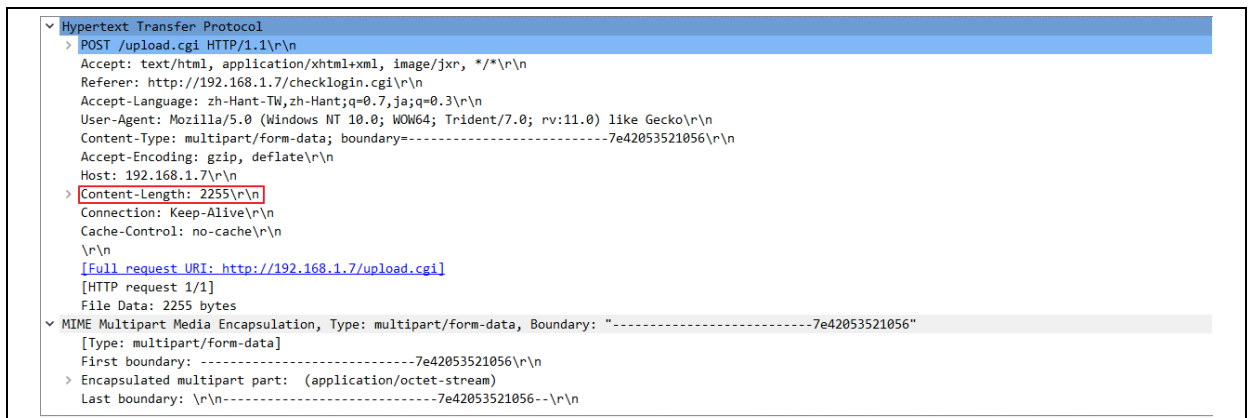
图 6 IE11 HTTP 头文件格式
