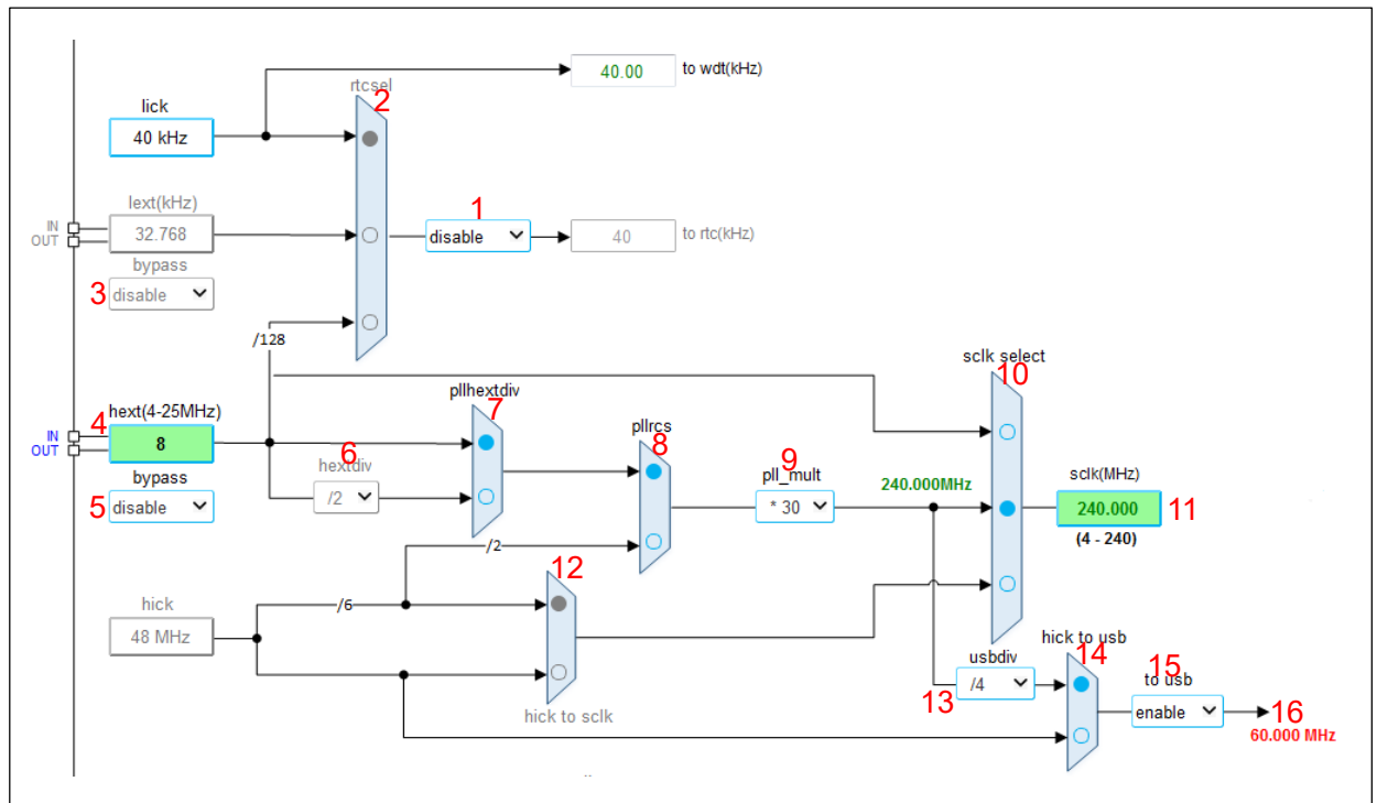
图 8. 时钟配置框
