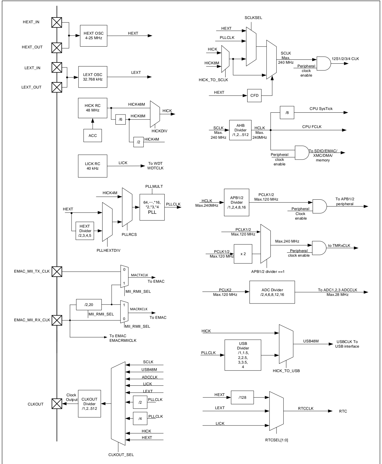
图 1. 时钟框图
