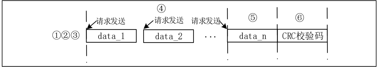
图 15 CRC 使用流程（轮询/中断方式）
