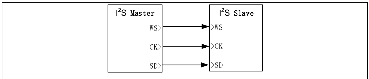
图 19 I 2 S 主发从收通信接线示意
