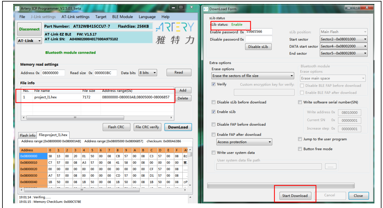
图 48. 终端用户烧录代码到 MCU
