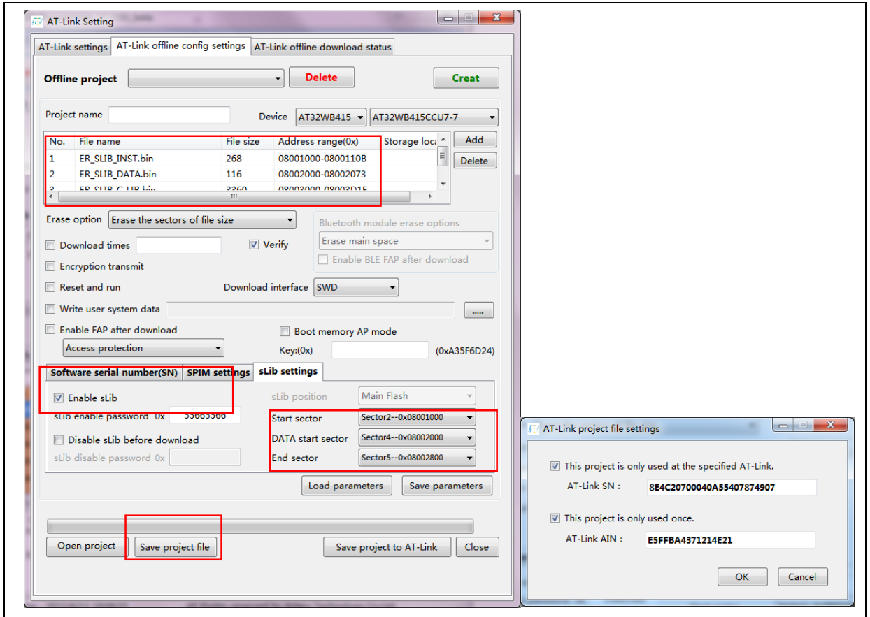
图 49. 制作离线项目工程
