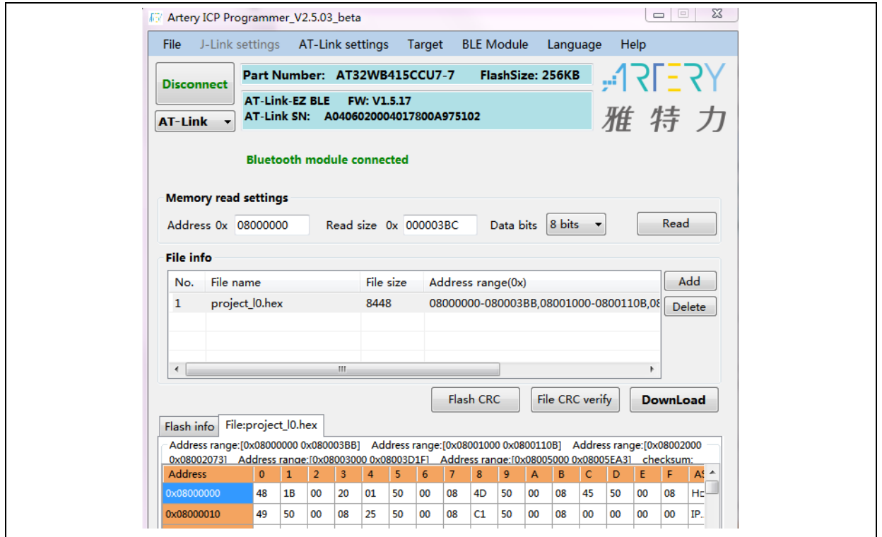
图 24. 配置 ICP Programmer
