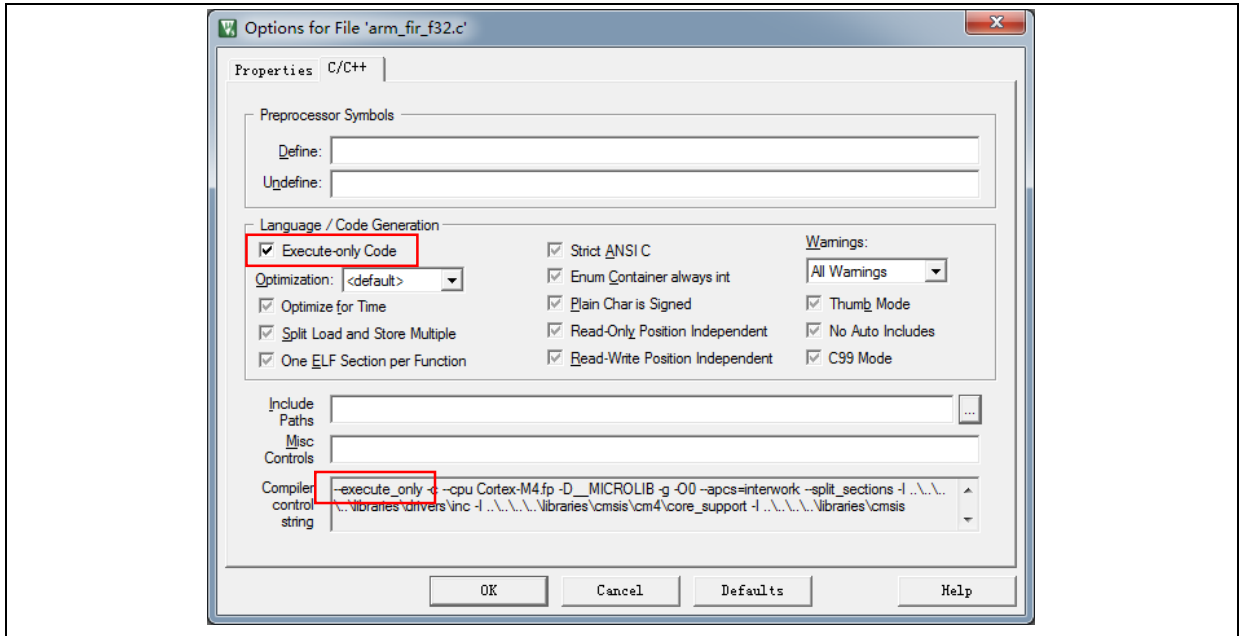
图 11. Keil 选择 Execute-only Code
