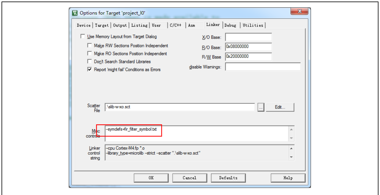
图 27. 设置 Keil Misc controls 选项
