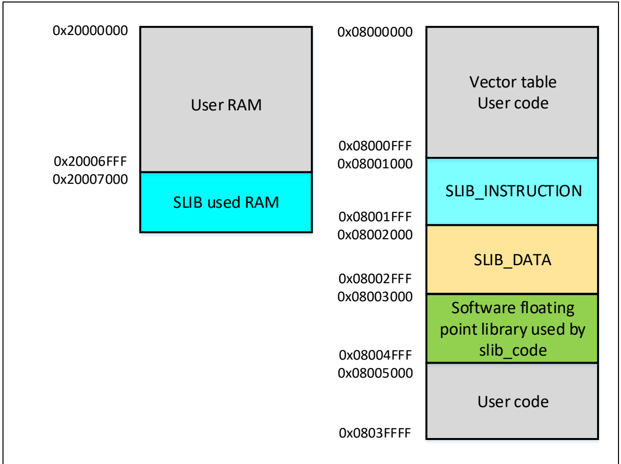
图 14. 范例程序的主闪存映像及 RAM 分区
