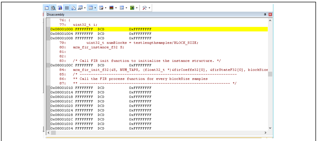
图 39. 代码查看
