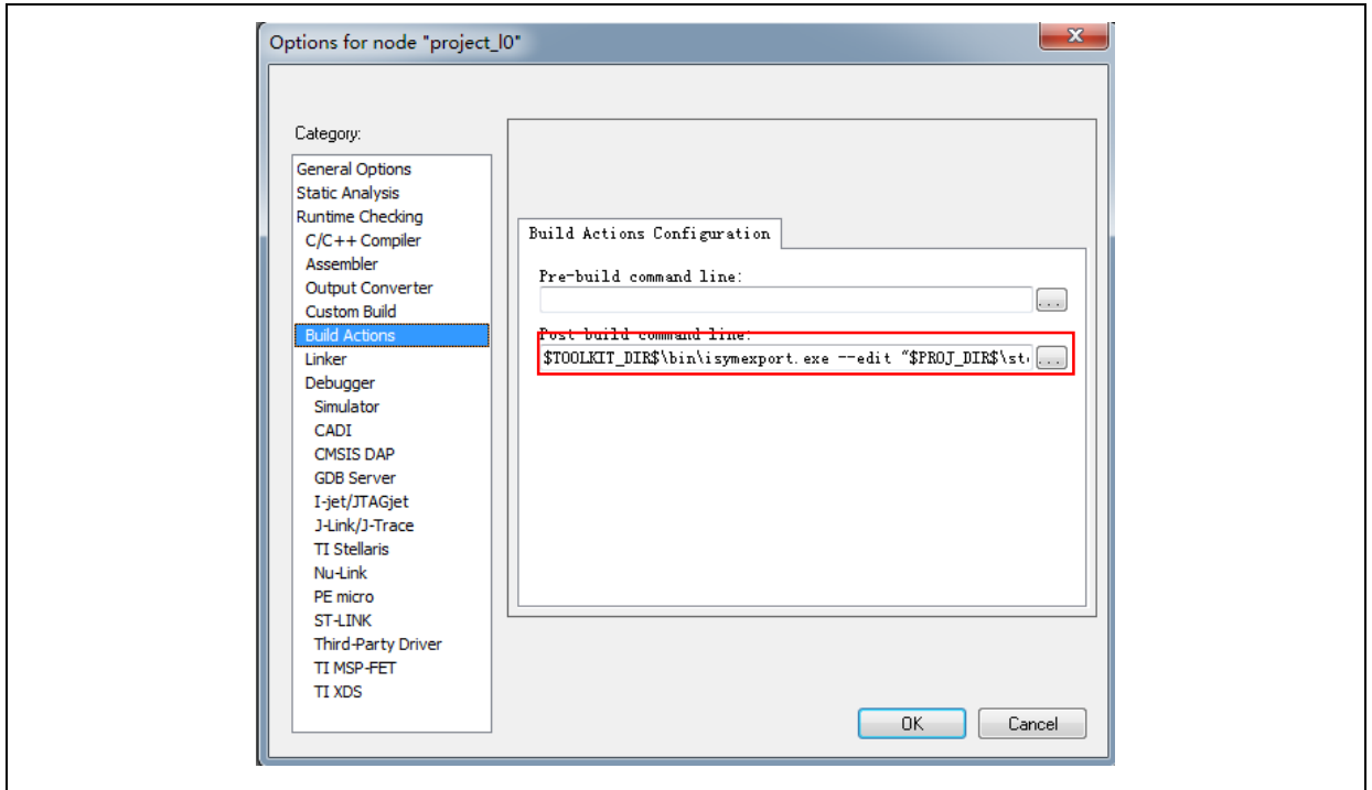
图 29. 设置 IAR Build Actions 选项
