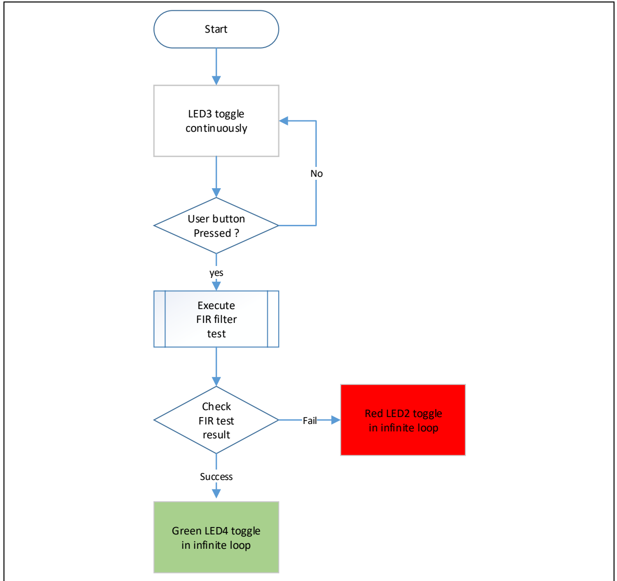
图 26. Project_L0 执行流程
