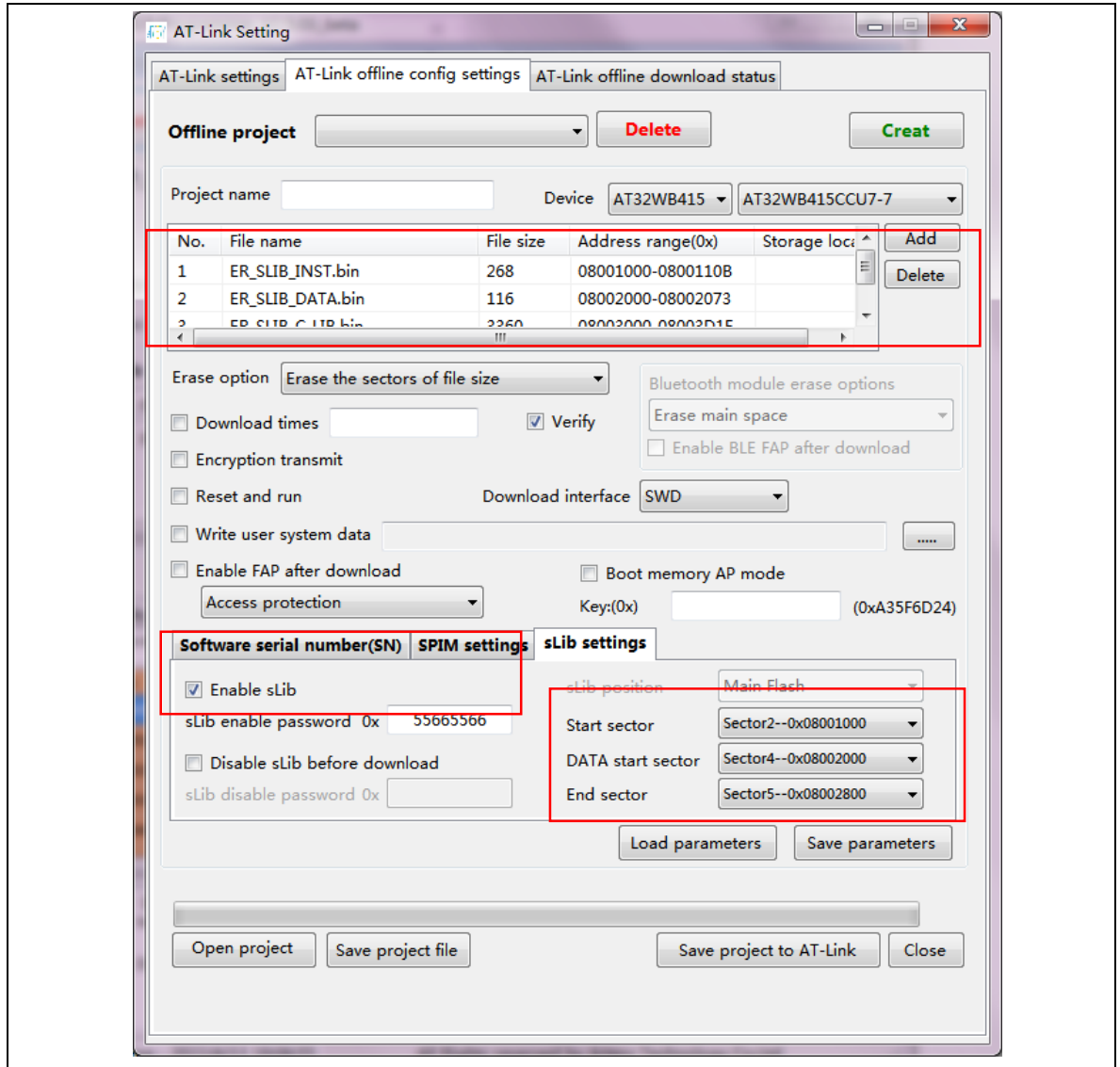
图 47. AT-Link 离线烧录到 MCU
