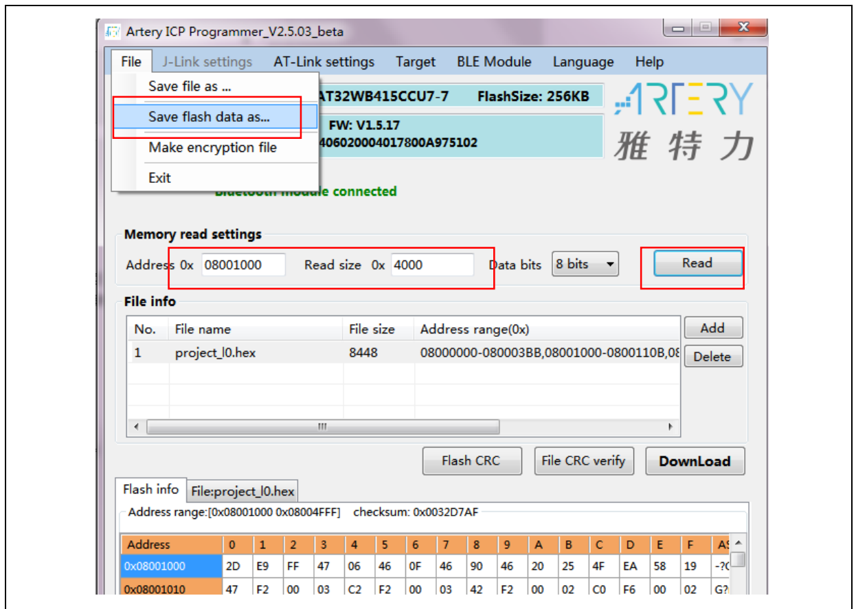
图 44. 保存 SLIB 代码
