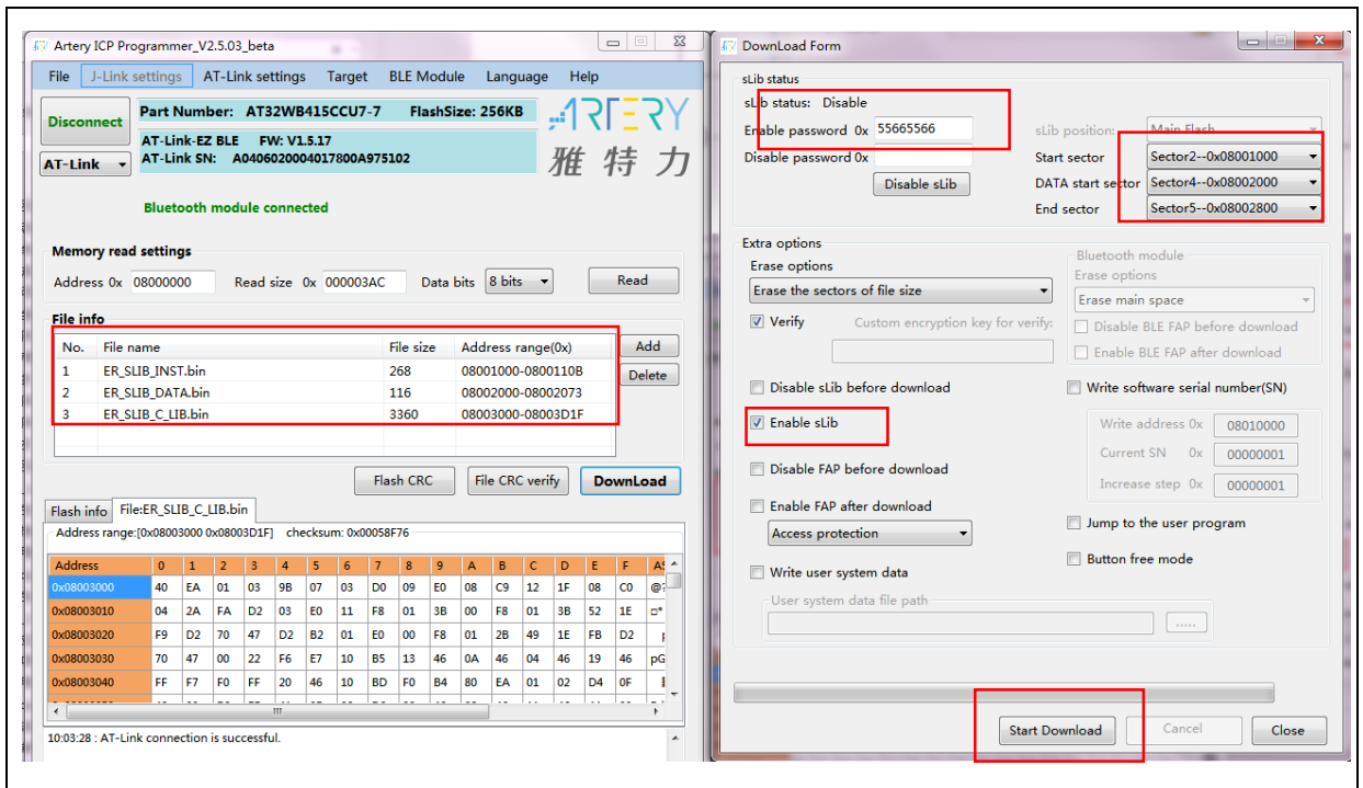
图 46. ICP 在线烧录 MCU
