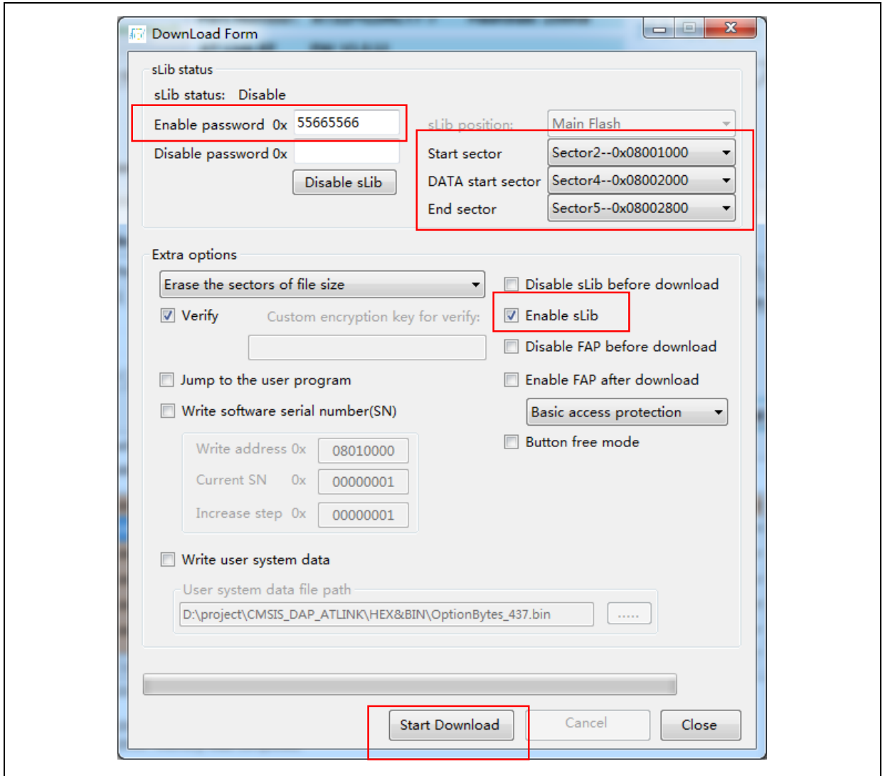
图 25. 设置下载选项参数
