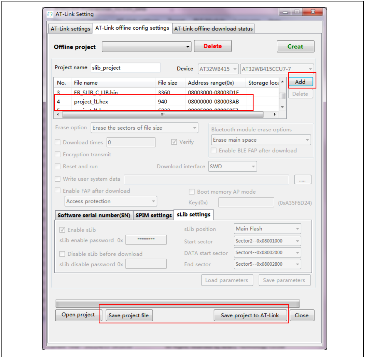
图 50. 添加项目文件
