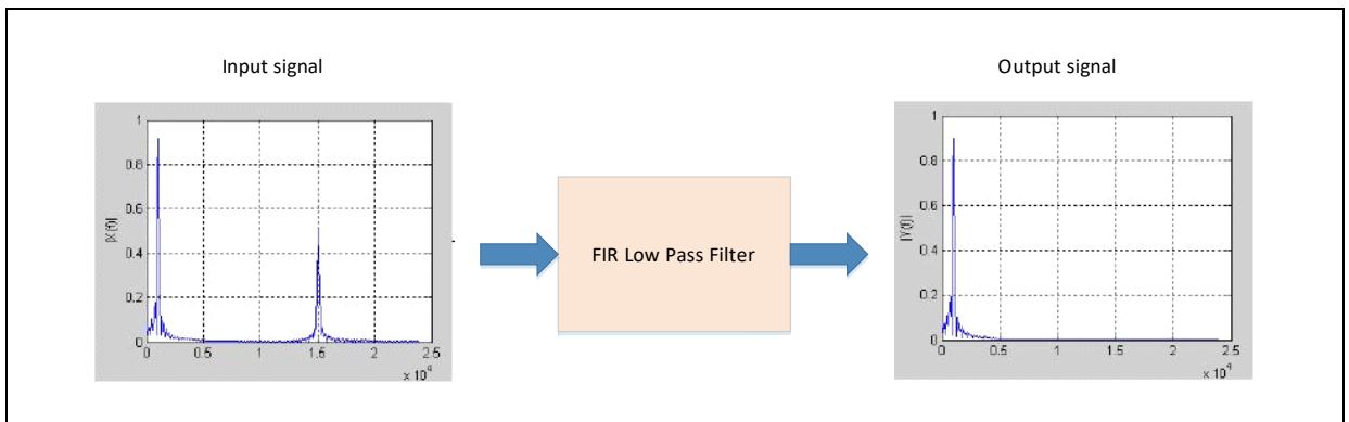
图 9. FIR 低通滤波器
