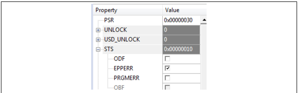
图 42. SLIB 写测试
