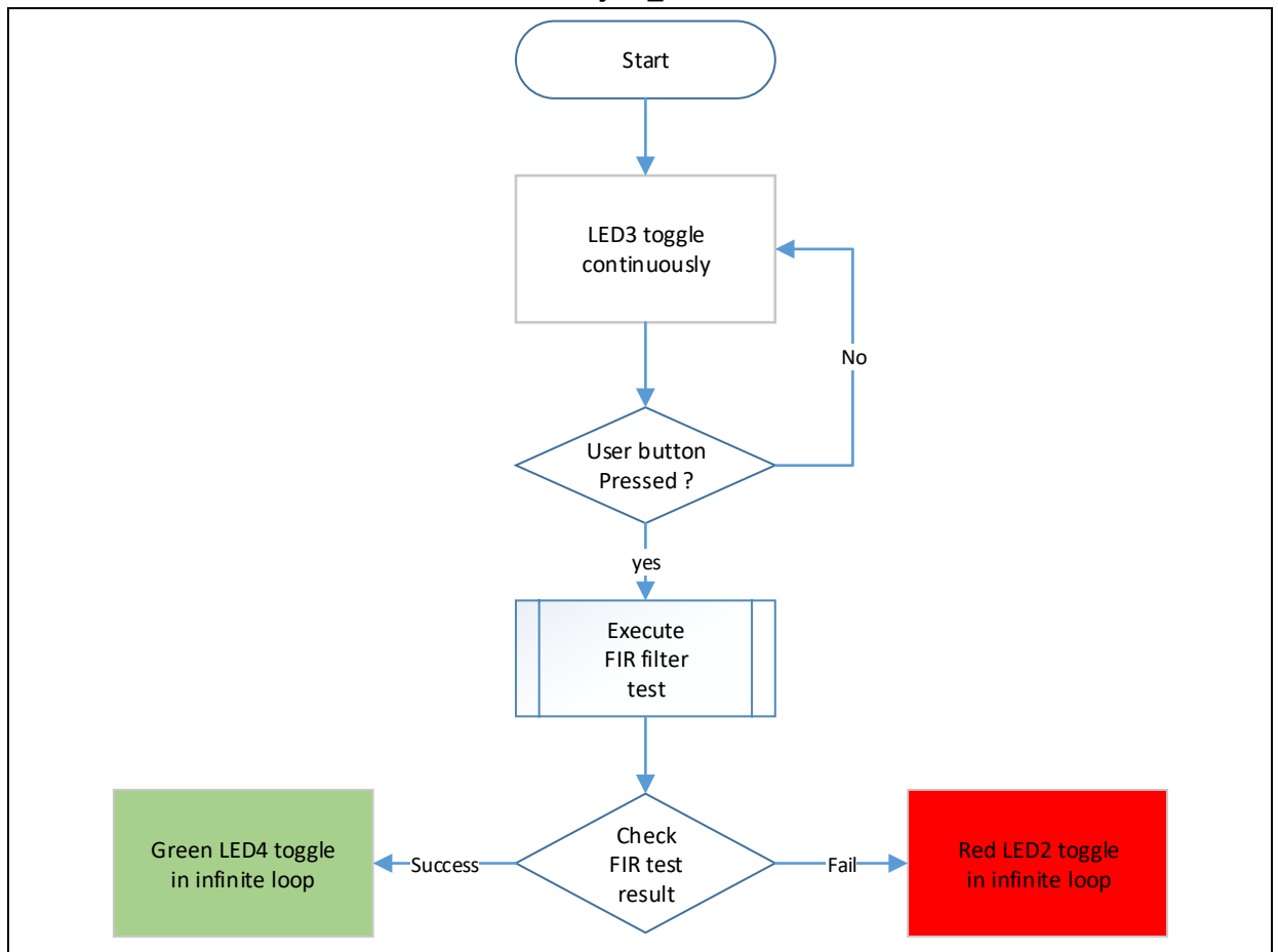
图 36. Project_L1 流程图
