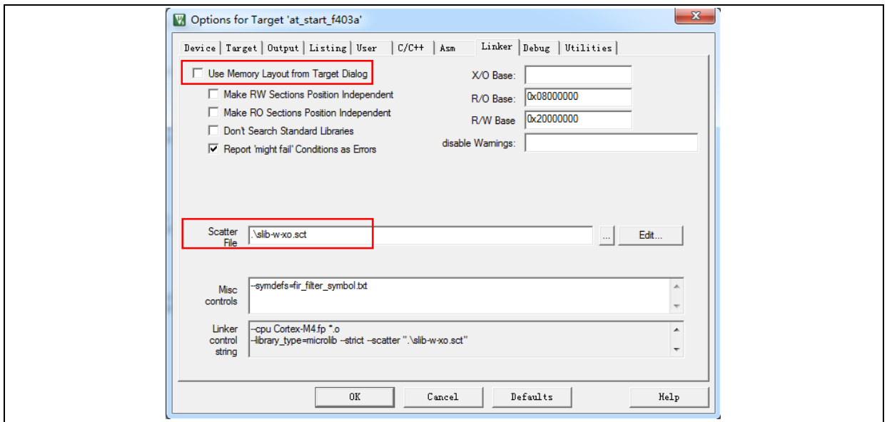
图 15. Keil 设置 Linker 窗口选项
