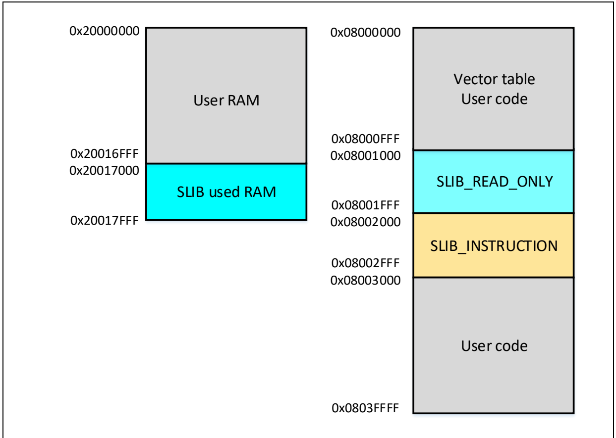
图 13. 范例程序的主闪存映像及 RAM 分区
