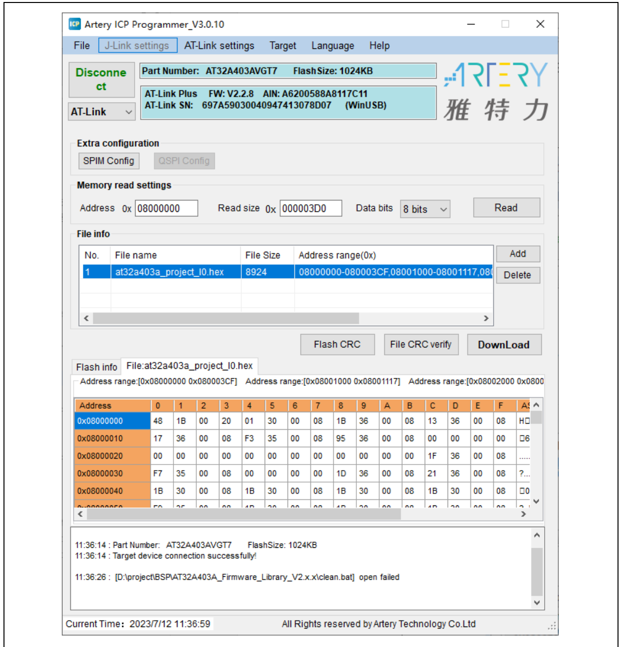
图 22. 配置 ICP Programmer
