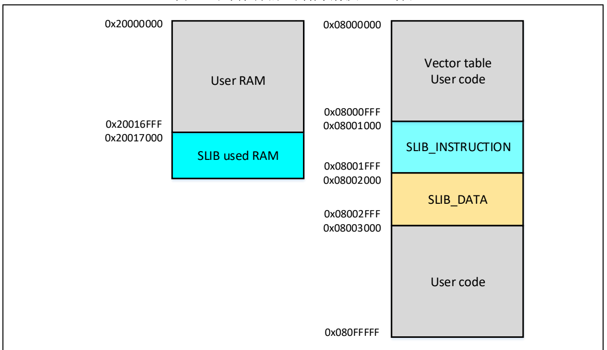
图 13. 范例程序的主闪存映像及 RAM 分区
