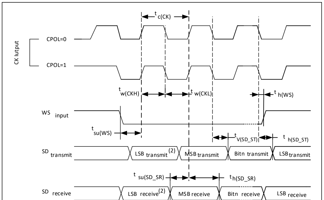
图 27. I 2 S 从模式时序图 (Philips 协议)
