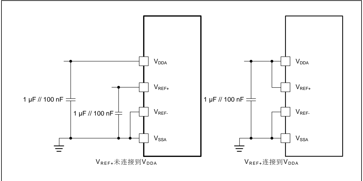
图 37. 供电电源和参考电源去耦线路（具有外部 V_{REF} 引脚封装）
