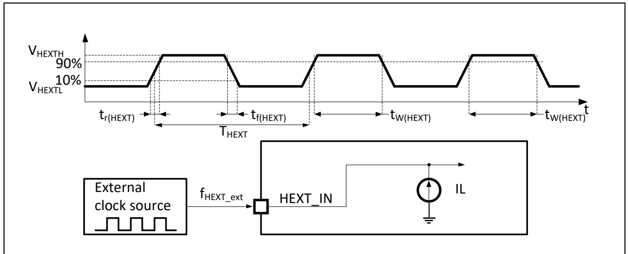
图 11. HEXT 外部时钟源交流时序图
