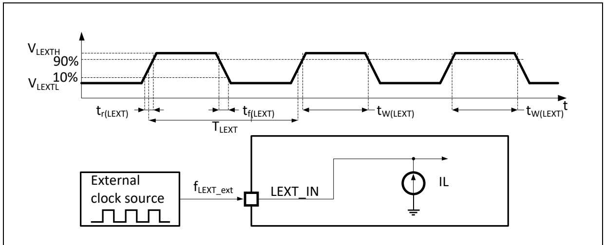
图 13. LEXT 外部时钟源交流时序图
