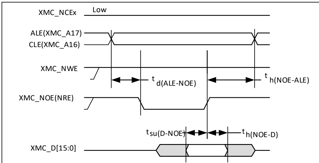
图 20. NAND 控制器读操作波形
