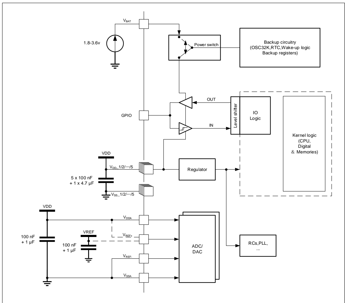
图 5. 供电方案
