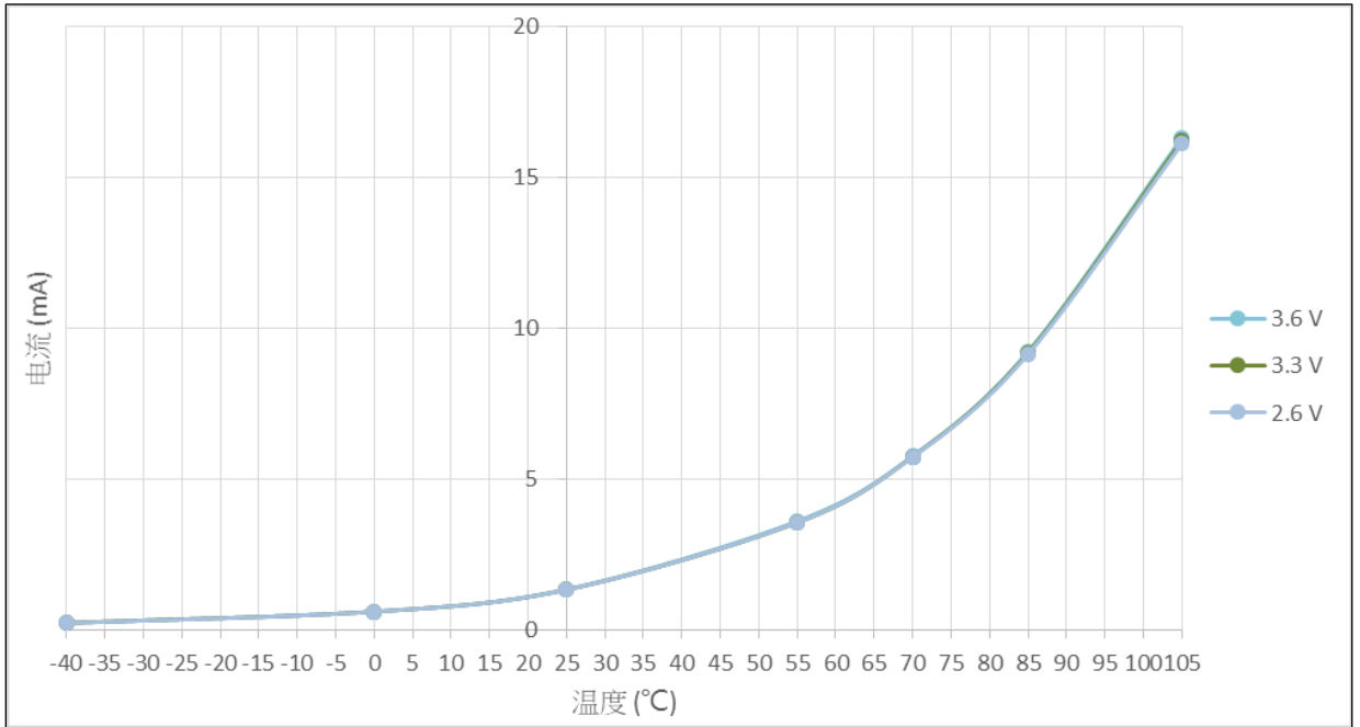
图 7. 深睡眠模式下的典型电流消耗在不同的 V_{DD} 时与温度的对比
