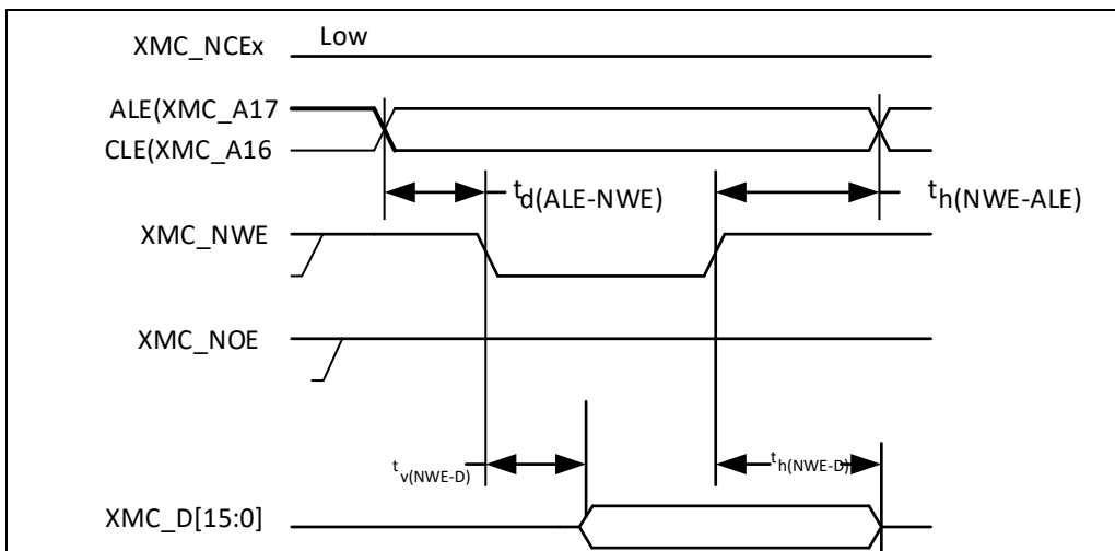
图 21. NAND 控制器写操作波形
