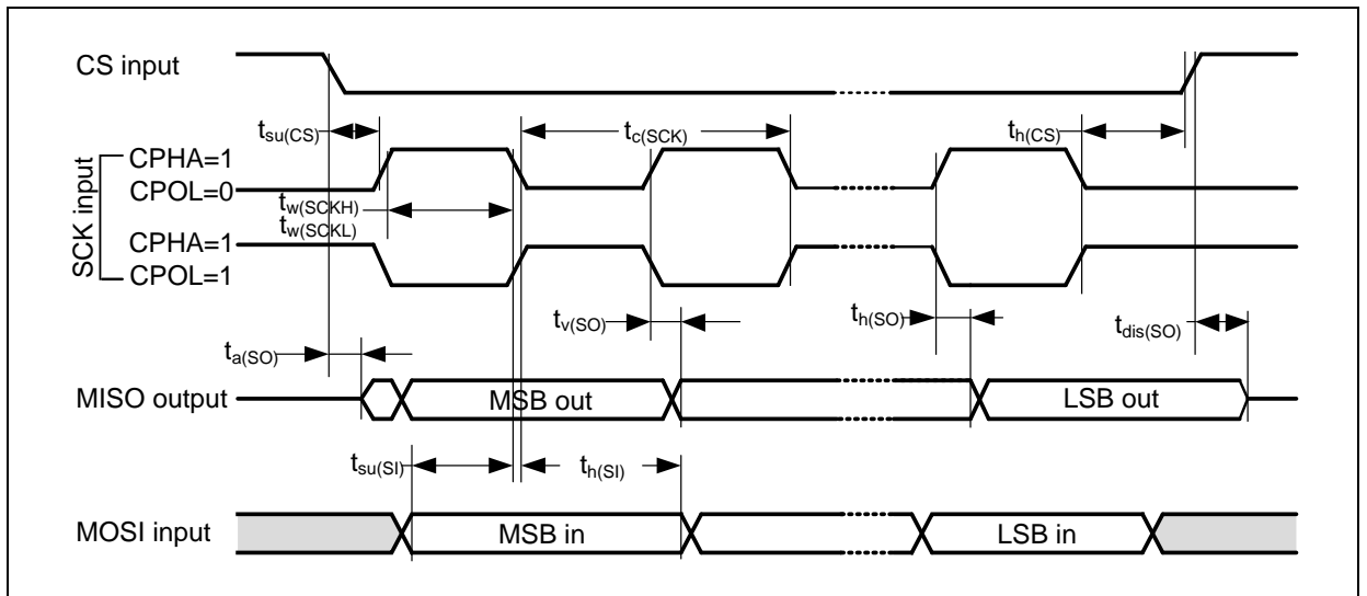
图 25. SPI 时序图 - 从模式和 CPHA = 1
