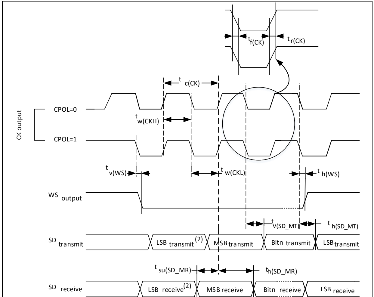
图 28. I 2 S 主模式时序图 (Philips 协议)
