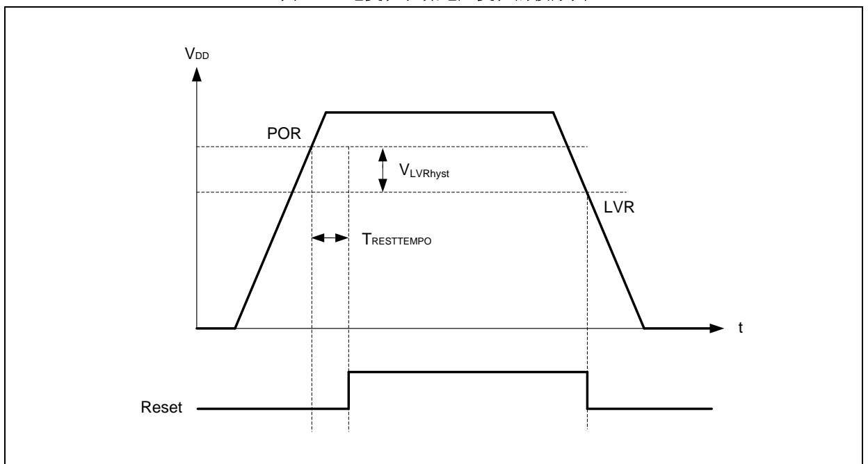
图 6. 上电复位和低电压复位的波形图
