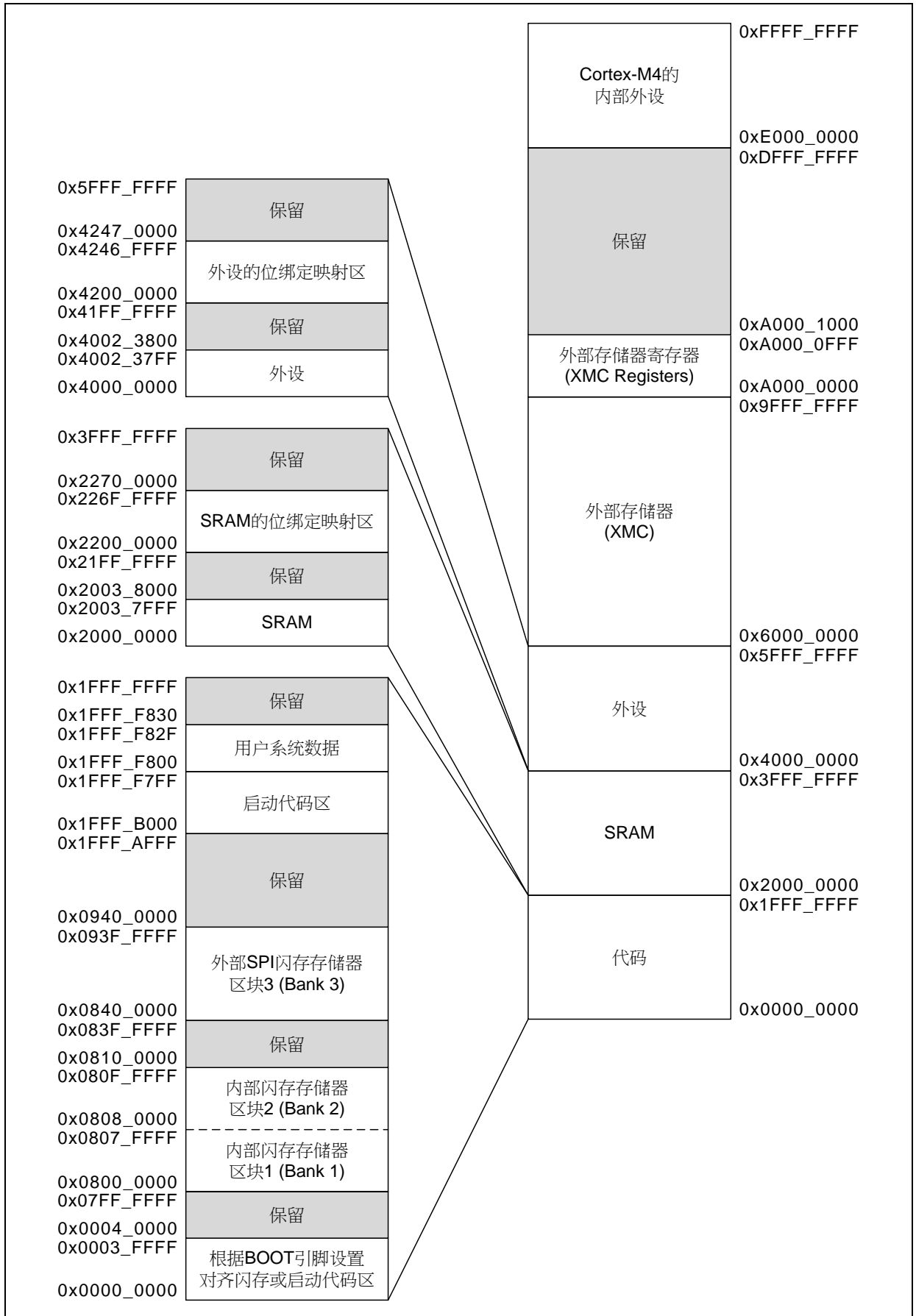
图 4. 存储器图
