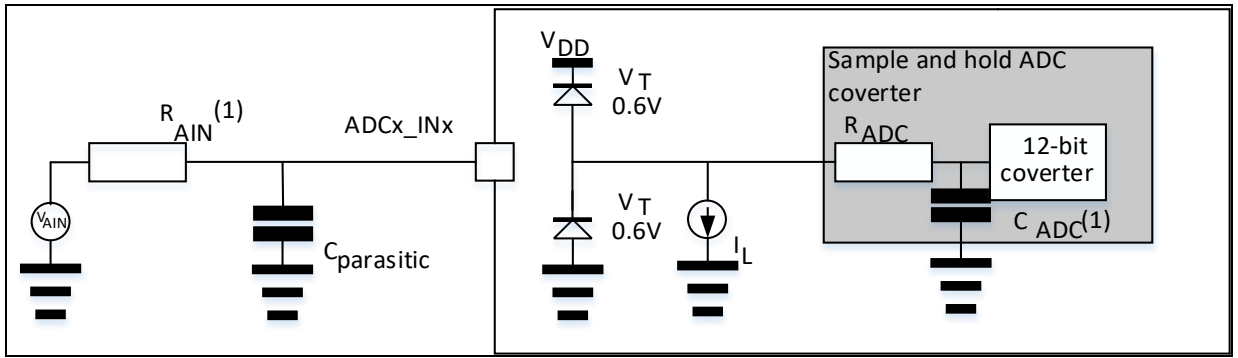
图 36. 使用 ADC 典型的连接图
