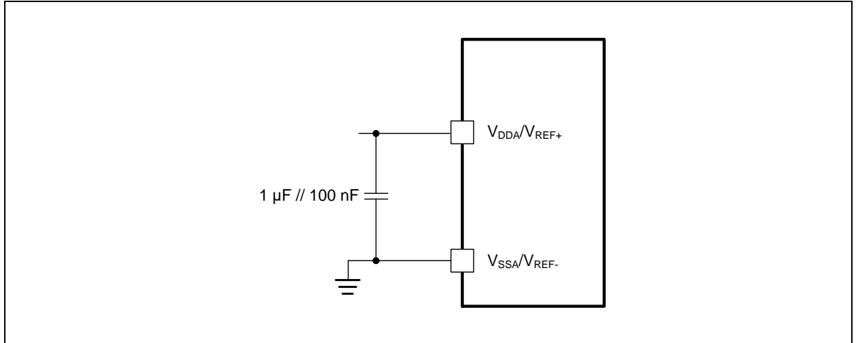
图 38. 供电电源去耦线路（无外部 V REF 引脚封装）
