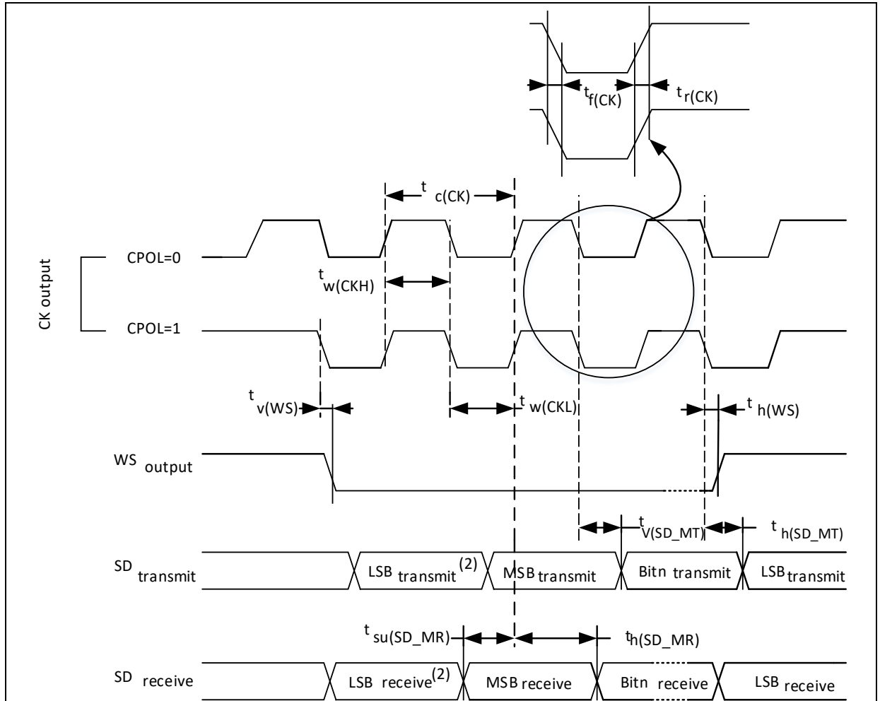
图 24. I 2 S 主模式时序图 (Philips 协议)
