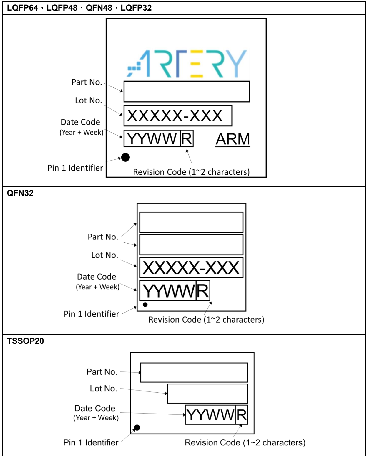
图 35. 丝印示意图
