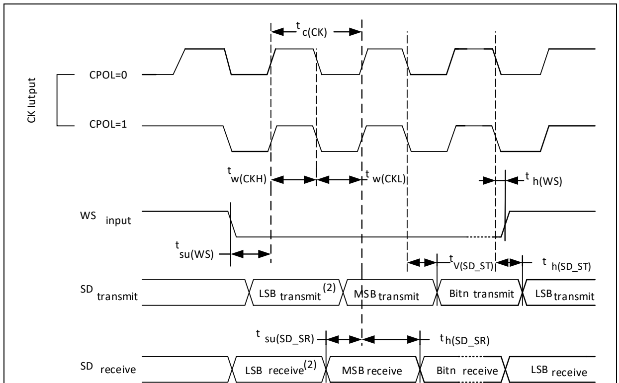
图 23. I 2 S 从模式时序图 (Philips 协议)
