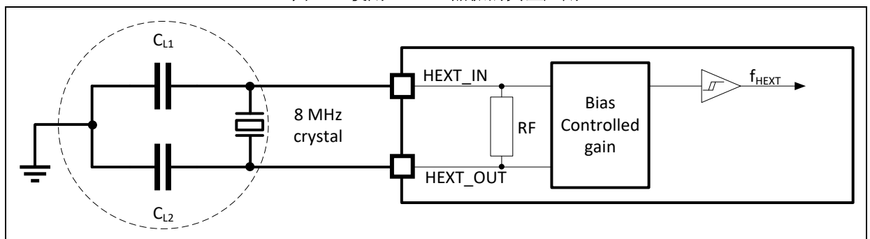
图 14. 使用 8 MHz 晶振的典型应用
